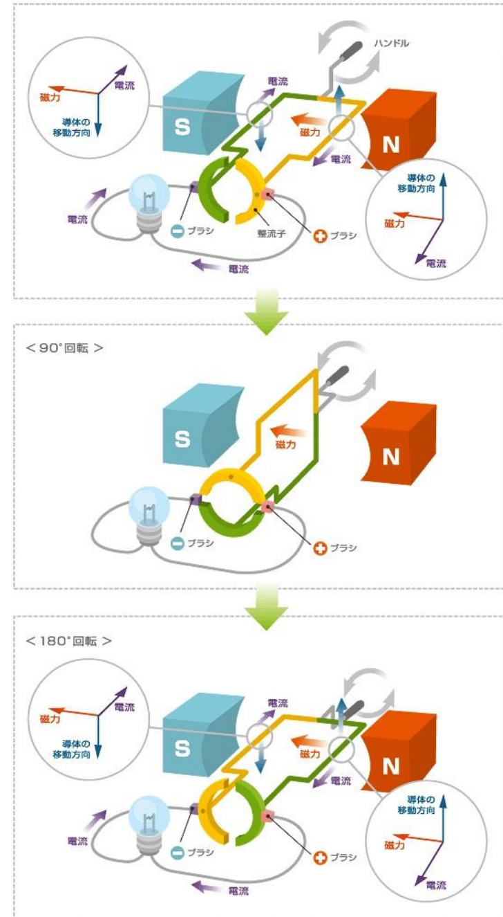
手回し発電機の仕組み
